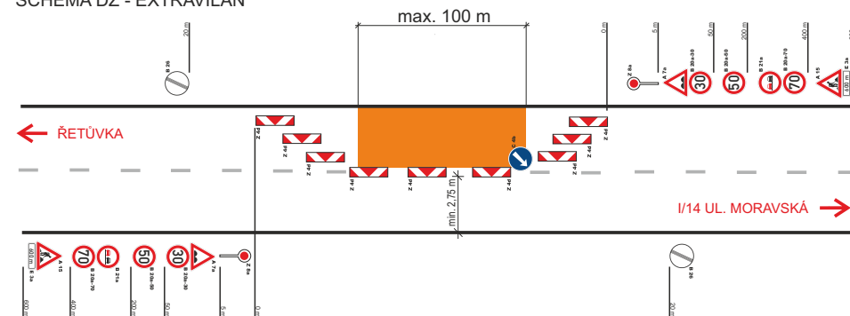
SCHÉMA DZ - EXTRAVILÁN
