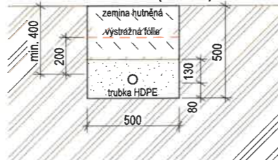
ŘEZ CHODNÍKEM (M 1:20)
