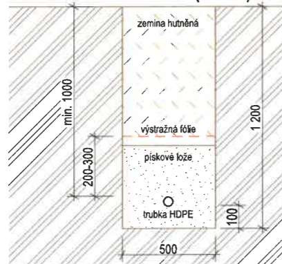
ŘEZ ZELENÝM PRUHEM (M 1:25)
