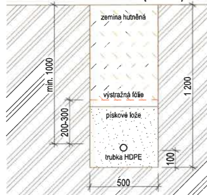
ŘEZ ZELENÝM PRUHEM (M 1:25)
